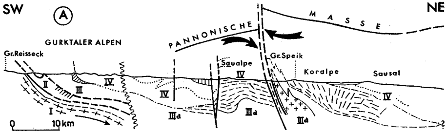
Abb. 2: Längsprofil durch die östlichen Zentralalpen, A—A
