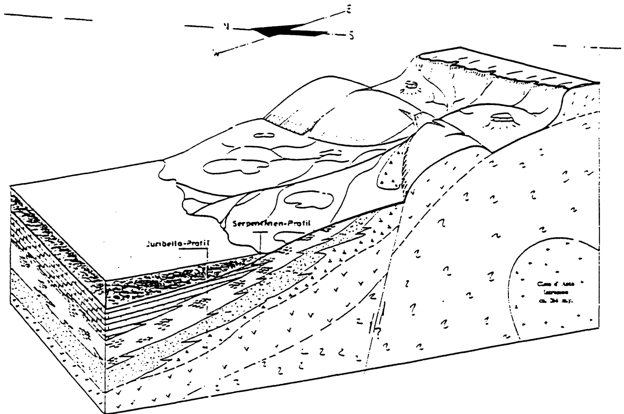
Abb. 3 Paläogeographisches Modell
