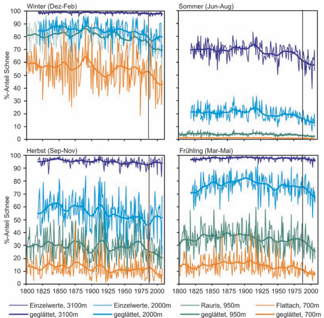
Abb. 26. Zeitreihen des Prozentanteils des Schnees am Gesamtniederschlag in den vier Jahreszeiten in Flattach (700m), Rauris (950m) und in Höhenlagen von 2000m und 3100m von 1800 bis 2007/08 (Einzelwerte und 30-jährig geglättet). Die vertikalen grauen Linien markieren den auf den Seiten 7 und 8 diskutierten Eintritt ins anthropogene Treibhausgaszeitalter in den 1980er Jahren.
