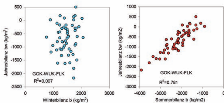
Abb. 37. Die Abhängigkeit der Jahresbilanz der drei Hauptgletscher des Sonnblickgebietes von der Winterbilanz (links) und von der Sommerbilanz (rechts). Stichprobe: 56 Bilanzjahre von Goldbergkees, Wurtenkees und Kleinfleijskees in den Jahren 1982-2008
