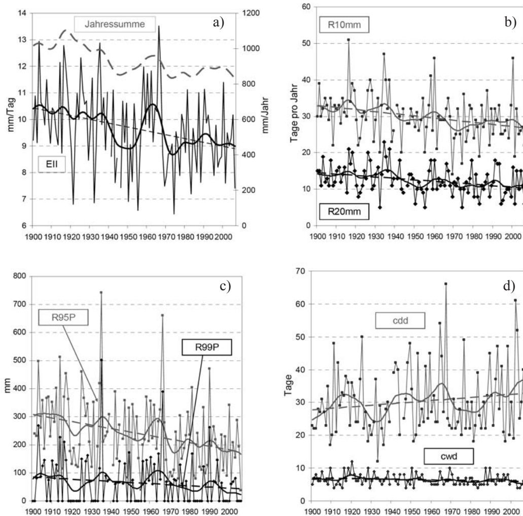
Abb. 41. Zeitreihen ausgewählter Climate Change Indizes in Flattach, Einzelwerte und 20jährig geglättete Kurvenverläufe und lineare Trends,
