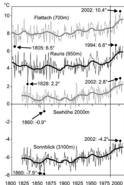
Abb. 20. Jahresmittel der Lufttemperatur in Flattach, Rauris, in den Hohen Tauern in 2000m und in 3100m Seehöhe (Sonnblick). Die dünnen Linien zeigen die Einzeljahre, die dicken sind 30-jährig geglättet. Talreihen 1800-2007, Bergreihen 1818-2007. Die kältesten und wärmsten Jahre der Zeitreihen sind als schwarze Punkte markiert. Die vertikale Linie in den frühen 1980er Jahren markiert die Wende vom natürlichen zum menschlich mit-beeinflussten Treibhausklima
