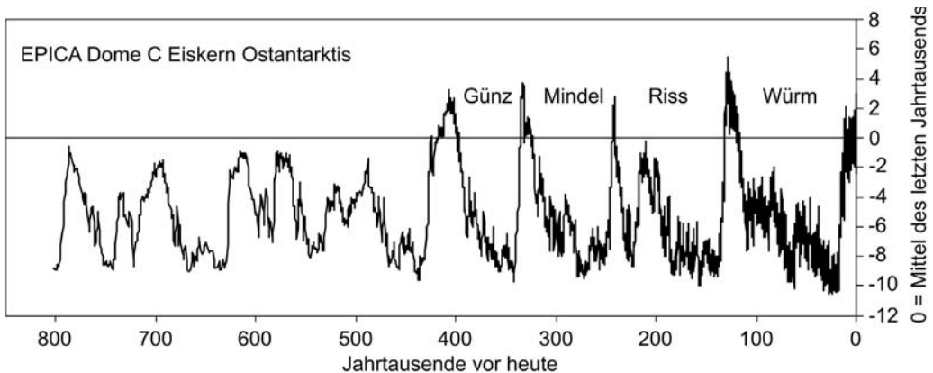
Abb. 13. 800.000 Jahre Temperaturschwankungen zwischen Eiszeiten und Zwischeneiszeiten, abgeleitet aus stabilen Isotopen ( ^{18}\text{O} oder \text{D} ) im Eis der Antarktis kalibriert an modernen Temperaturdaten. (EPICA community members, 2004)
