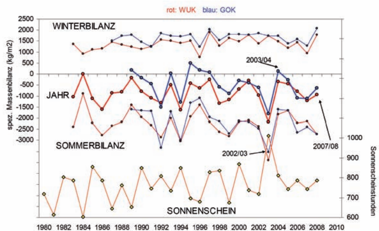
Abb. 36. Zeitreihen der Massenbilanzen für das Wurtenkees (rot, 1982-2008) und für das Goldbergkees (blau, 1988-2008). Oben: Winterbilanzen, unten: Sommerbilanzen, Mitte: Jahresbilanzen. In orange zum Vergleich die Sonnenscheindauer in der Ablationsperiode (Mai-September), gemessen auf dem Sonnblick
