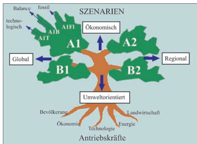
Abb. 3: Die Szenarienfamilie des IPCC. Quelle: IPCC (2000), mit freundlicher Genehmigung
