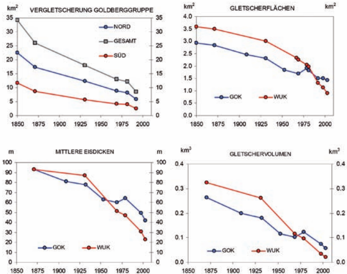
Abb. 32. Kartometrische Zeitreihen der Vergletscherung der Goldberggruppe. Links oben: Flächen aller Gletscher der Gruppe, unterteilt nach nördlich und südlich des Alpenhauptkamms 1850-1992 (Böhm, 1992) Rechts oben: Flächen von Wurtenkees (WUK) und Goldbergkees (GOK) 1850-2003 Unten links: Mittlere Eisdicken 1871-2003, unten rechts: Gletschervolumina 1871-2003 (Binder, 2008, Binder et al., 2009 kombiniert mit Böhm et al., 1983)
