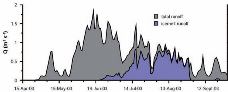
Abb. 38. Tägliche Abflussmengen (in m^3 pro Sekunde) der Pegelmessstelle Goldbergkees. Grau hinterlegt ist der gesamte Abfluss, blau hinterlegt ist die Eisschmelze. Im Mai und Juni ist das Abschmelzmaximum des Schnees zu erkennen, August 2003 war der Anteil der Eisschmelze nahe 100%. Quelle: G. Koboltschnig, 2007
