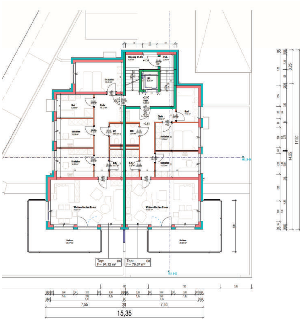
Abb. 10: Projekt „Wohnen im Grünen“ – Grundriss 01 OG [18]
