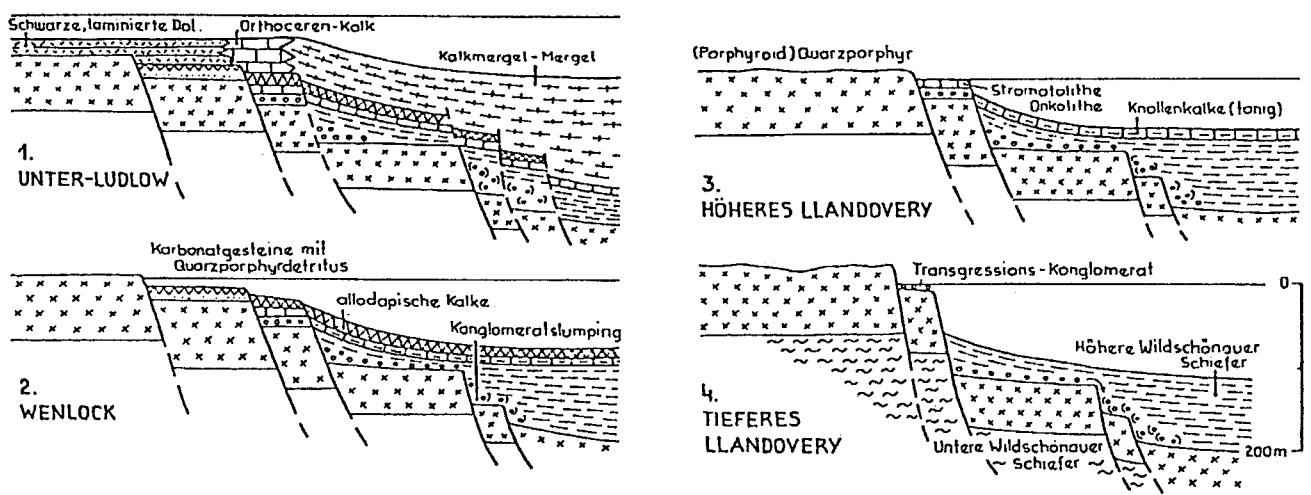
Abb. 6. Eine synsedimentäre Bruchtektonik führte ab dem tieferen Silur zu Faziesdifferenzierungen in der westlichen Grauwackenzone (nach H.MOSTLER, 1970). (Aus A.TOLLMANN, 1977).
