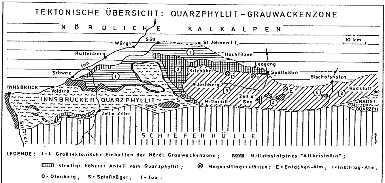
Abb. 4. Großtektonische Skizze des Westabschnittes der Grauwackenzones (aus H. MOSTLER, 1973).
