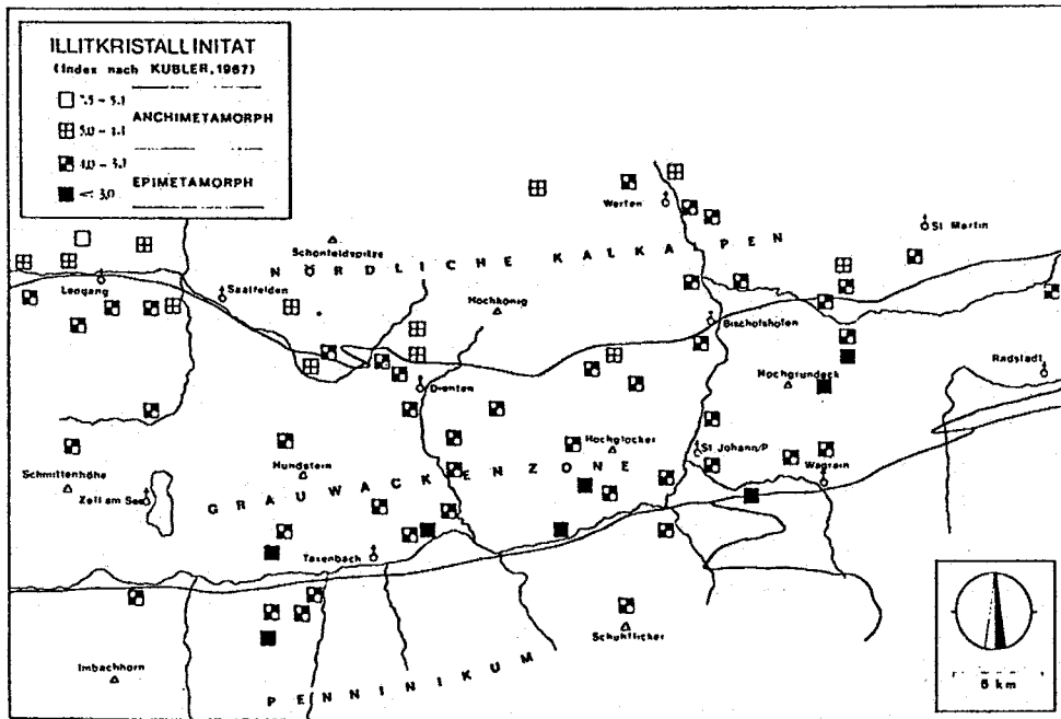
Abb. 11. Verbreitung der Illit-Kristallinität (KÜBLER-Index), Grenze Epi-/Anchizone: 4.0mm = 0.25°δ2θ, Grenze Anchizone/Diagenese: 7.5mm = 0.42°δ2θ (aus D.BECHTOLD et al., 1981).
