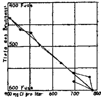
Abb. 5. Graphische Darstellung des Verhältnisses zwischen der Tiefe eines Brunnens und dem Chlorgehalt des gelieferten Wassers. Durch Zuspופן mit Beton wurde der Chlorgehalt vermindert.
