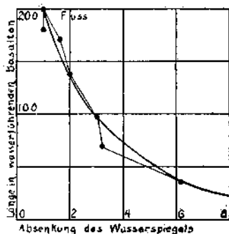
Abb. 6. Graphische Darstellung des Verhältnisses zwischen der Größe der wasserliefernden Oberfläche innerhalb eines Brunnens und des Sinkens des Wasserspiegels unter gleicher Wasserentnahme. Durch Zustopfen mit Beton war das Sinken gesteigert, und die Ergiebigkeit des Brunnens vermindert.
