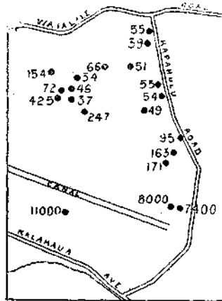
Abb. 7. Geographische Verteilung von Chlor (mg Chlor pro Liter im isopiezischen Bezirke I.
