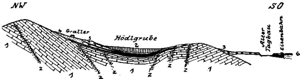
Abb. 2. Geologischer Schnitt durch die Hödlgrube. Schwarz: Kohle; z: Zerrüttungsstreifen, z. T. mit Verwerfungen oder Schichtenknickungen verbunden; 1 = Unterdevon; 2 = Ausgekohlte Oberbank samt Hangendmittel; 3 = Gehängelehm; 4 = untermiozäne Sande; 5 = untermiozäne Tegel; 6 = junge Schotter der Talaue (Gradnerbach).
