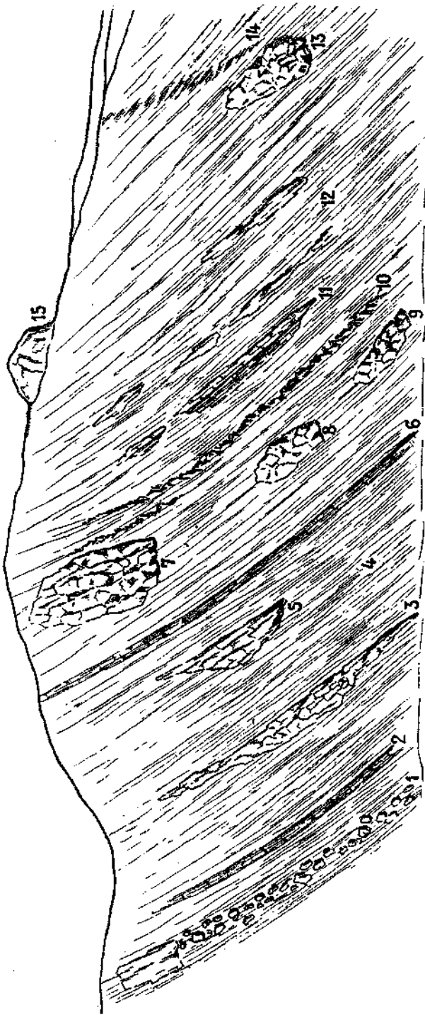
Fig. 1. Werfener Schiefer mit eingepreßten Neokalkblöcken in Valea seaca bei Kimpolung, Bukowina.
