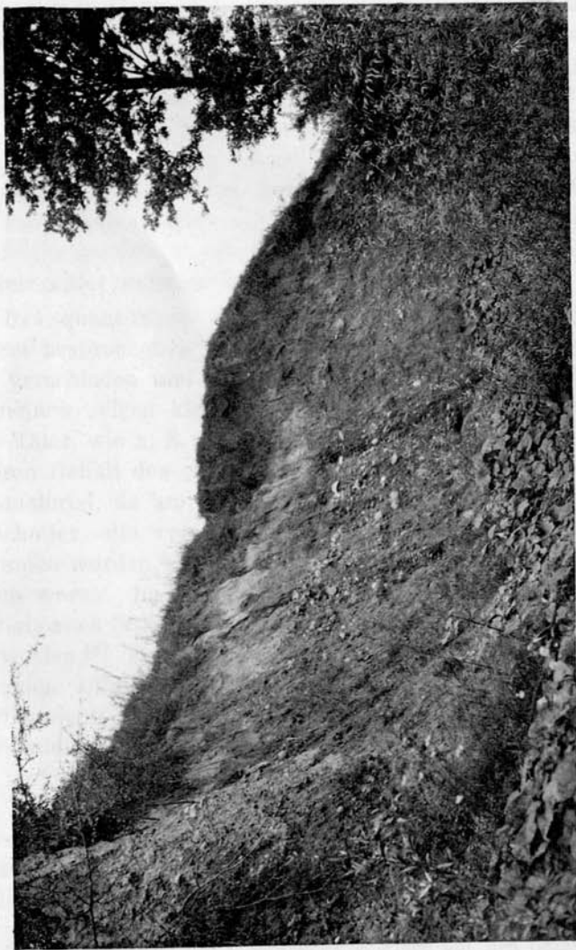
Mischschotter am linken Ufer eines Seitenbaches des Dunajec am unteren Ende von Tworkow bei Czchów im polit. Bezirke Brzesko. (Verf. phot. September 1908).
