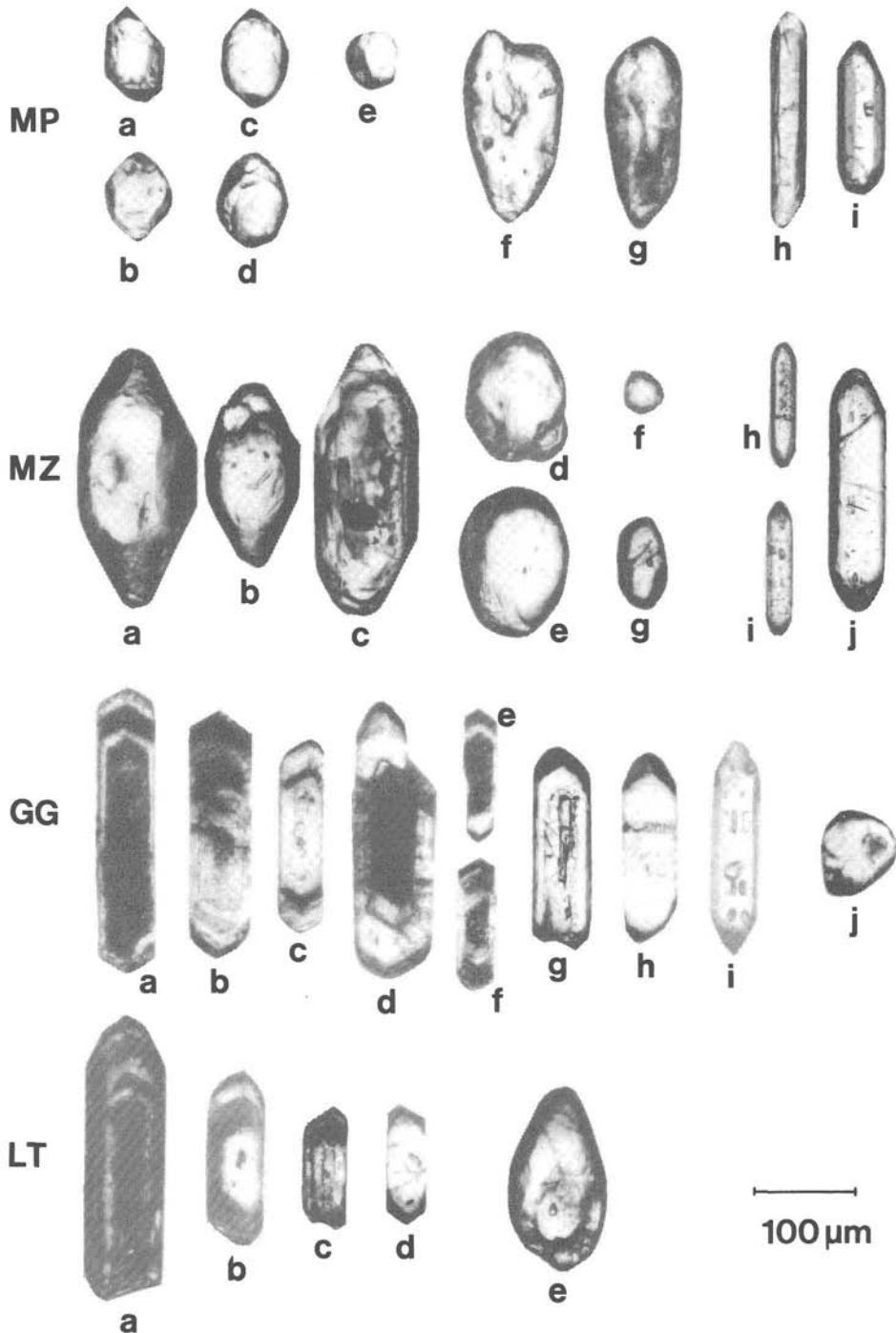
Tafel 1: Charakteristische Zirkone aus den Migmatischen Plagioklasgneisen (MP), Migmatischen Zweiglimmergneisen (MZ), Göb-Granitoiden (GG) und dem Leukotonalit (LT).
