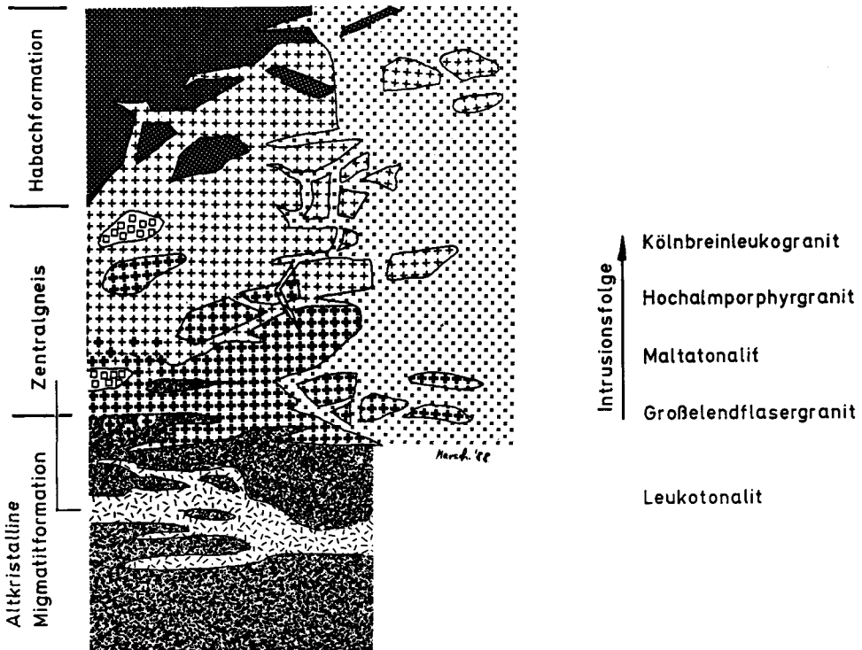
Abb. 3: Schematisierter Schnitt durch den Intrusionsverband im Untersuchungsgebiet: Die Zentralgneiseintrudieren im Liegenden und im Hangenden Gesteine des Alten Daches. Die Intrusionsabfolge der Zentralgneise weist einerseits kontinuierliche Gesteinsübergänge (Schlierenmigmatite), andererseits scharf begrenzte Intrusionskontakte (Schollenmigmatite) auf. Schollen der älteren Zentralgneise zeigen mit wachsender Entfernung vom Intrusionskontakt eine zunehmende Entfestigung und Zurundung. Die Gesteinsignaturen entsprechen Abb. 2.
