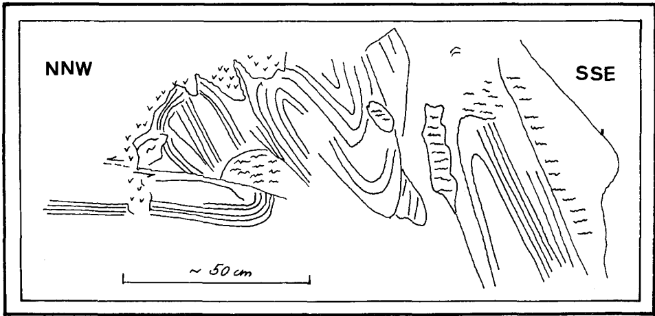
Abb. 4: Bachaufschluß 250 m SW Infangalm in 680 m Höhe, 180 cm über dem Bachbett. Wechsellagerung schiefriger und kieseliger Schichten (Mangan-Strubbergschiefer) im Liegenden der Strubbergbrekzie; aufrechte Serie, Faltenwurf mit NNW-Vergenz und sekundärer nordvergenter Zerschering eines Faltenschenkels (Tennengebirgstirolikum).
