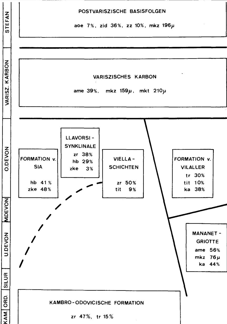
Abb. 7: Lithostratigraphisches Modell der klastischen Schichtfolgen mit hochsignifikanten durchgezogenen Trennlinien (Irrtumswahrscheinlichkeit 0.5%) und signifikanten strichlierten Trennlinien (Irrtumswahrscheinlichkeit 2.5%) unter Angabe der Mittelwerte der wichtigsten Unterscheidungsmerkmale (Abkürzungen s. Tab. 1).
