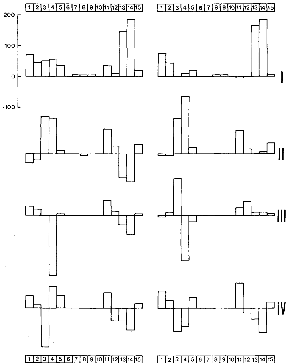
Abb. 5: Factor scores der nicht rotierten und rotierten Faktoren I—IV im Q-Modus. 1 = opak, 2 = Apatit mit Einschlüssen, 3 = Apatit ohne Einschlüsse, 4 = Zirkon idiomorph, 5 = Zirkon gerundet, 6 = Zirkon zonar, 7 = Turmalin idiomorph, 8 = Turmalin gerundet, 9 = TiO 2 -Minerale, 10 = Granat, 11 = Hornblende, 12 = Zoisit-Klinozoisit-Epidot, 13 = maximale Korndurchmesser Zirkon, 14 = maximale Korndurchmesser Turmalin, 15 = Karbonatgehalt.
