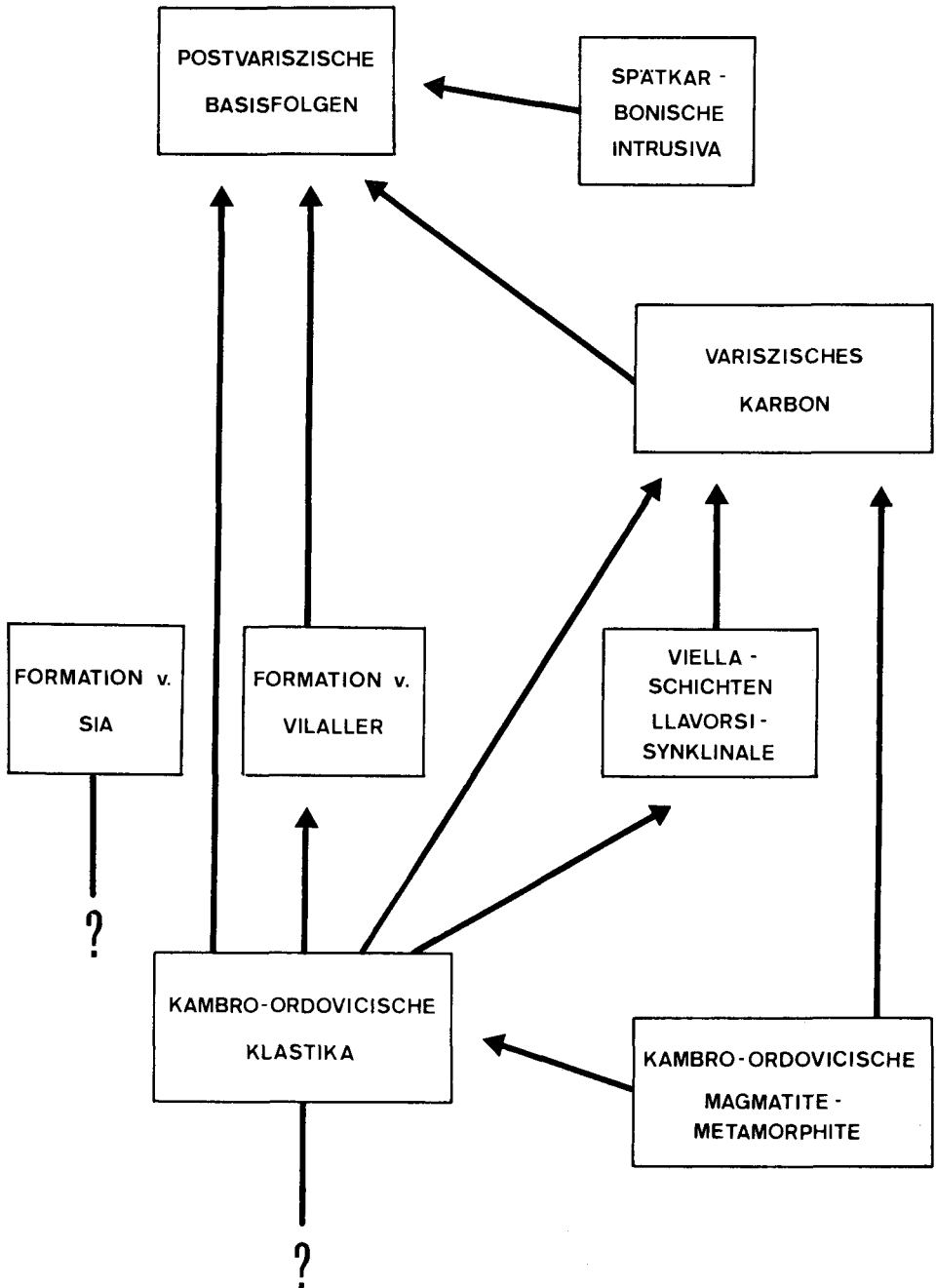
Abb. 8: Rekonstruktion der Liefergebiete der klastischen Schichtfolgen nach dem lithostratigraphischen Modell in Abb. 7.
