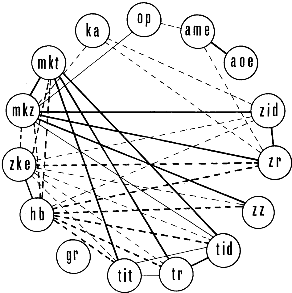
Abb. 6a: R-Modus Cluster-Diagramm von 84 Proben aus präkarbonischen Klastika mit 15 Variablen (Abkürzungen s. Tab. 1). Signifikanz-niveau 99% (dicke Linien) und 95–99% (dünne Linien). Signifikant negative Korrelationen sind strichliert gezeichnet.
