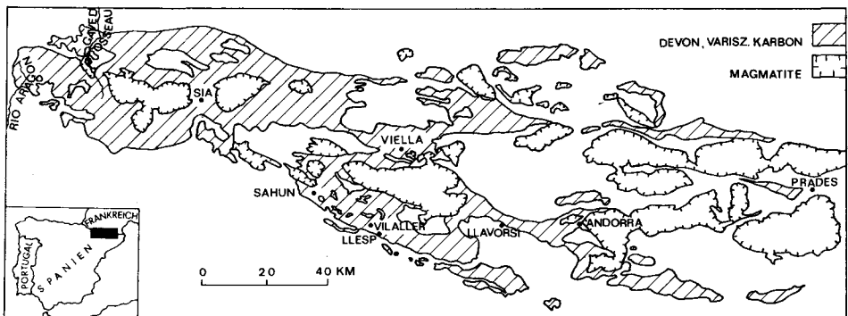
Abb. 2: Geologische Übersichtskarte des Untersuchungsgebietes (nach ZWART 1972).
