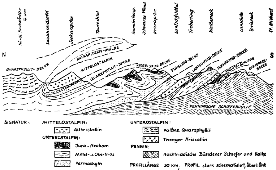
Abb. I Schematisches Sammelprofil durch die Radstädter Tauern
